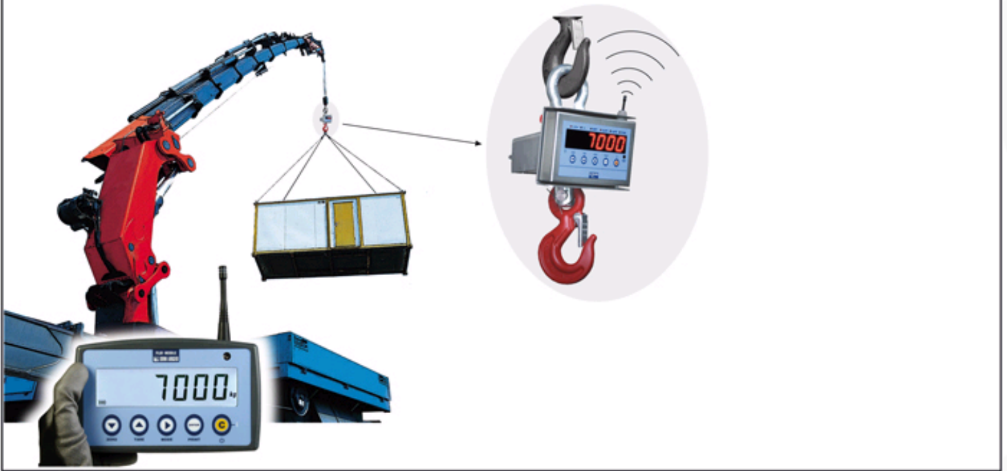
DFWPM: Peer-to-peer Fernanzeige mit einer Waage.
