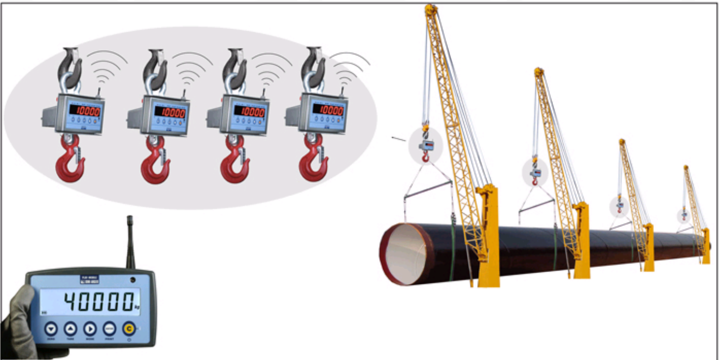
DFWPM: Fernanzeige für mehrere Waagen.
